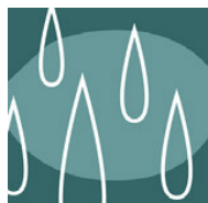
Bara naturlig försurning
